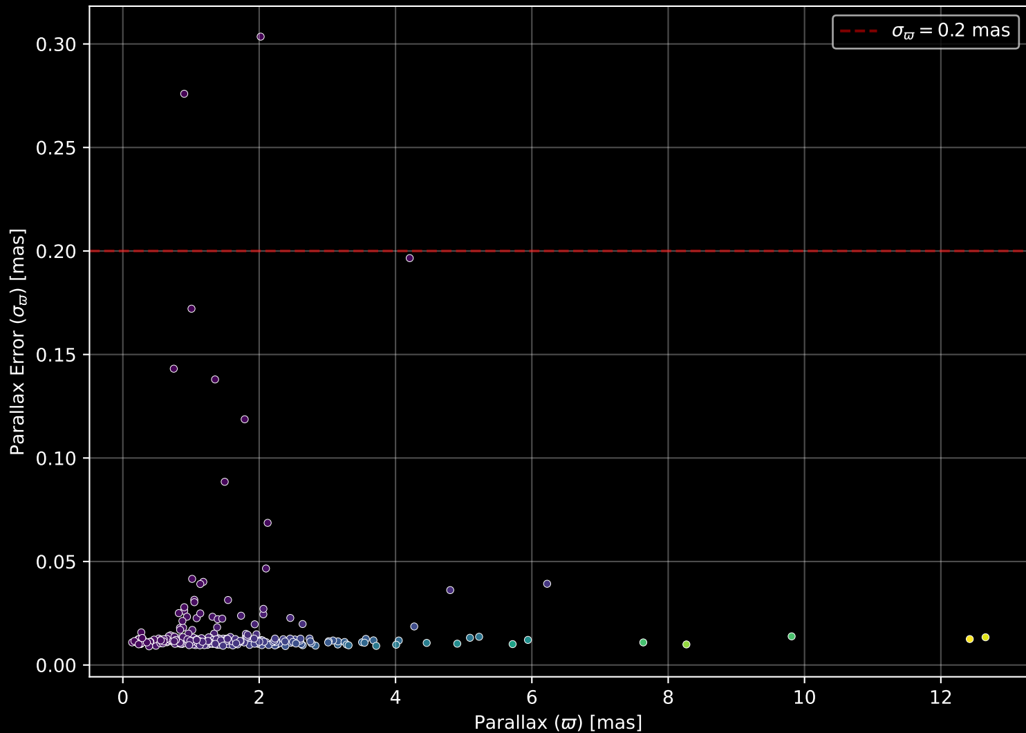
GALAH DR4 Field: [887] Parallax Quality (n= 290)
