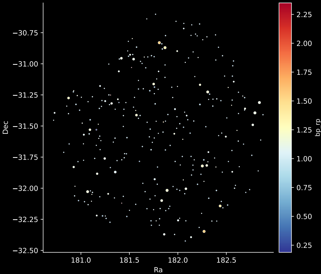
GALAH DR4 Field: [887] Stars: 290
