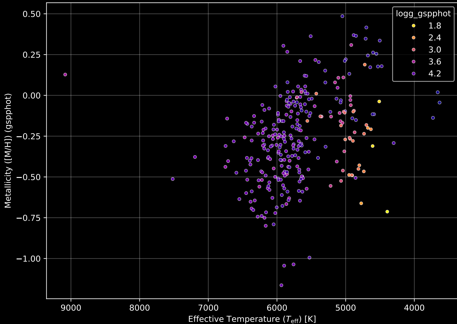
GALAH DR4 Field: [887] Stellar Population Parameters (n= 290)
